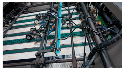
枚葉印刷機 給紙部
